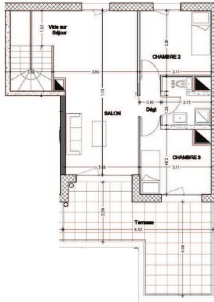
Plan étage
